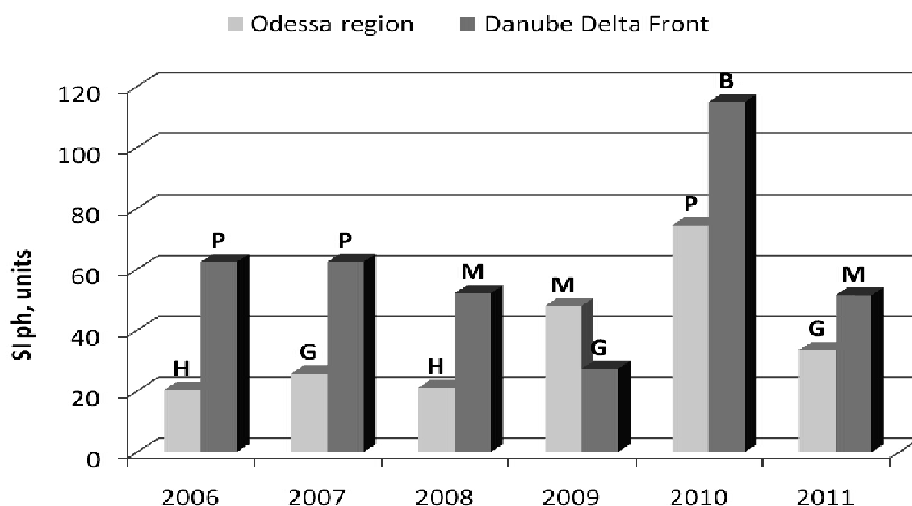
Fig. 6 Comparative characteristics of ESC between Odessa region and the Danube Delta Front: H – High; G – Good; M – Moderate; P – Poor; B – Bad Рис. 6 Сравнительная характеристика экологических статус классов (ESC) Одесского региона и авандельты Дуная: H – высокий; G – хороший; M – средний; P – недостаточный; B – плохой
