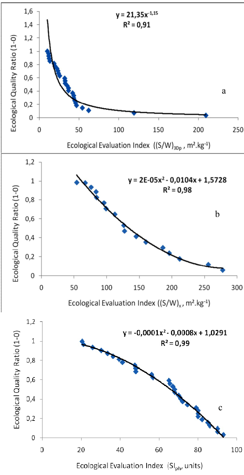
Fig. 2 Approximations of the different EEI to the EQR's scale: a – (S/W)_{3Dp} ; b – (S/W)_x ; c – SI_{ph} Рис. 2 Аппроксимация различных индексов экологической оценки (EEI) к шкале относительного экологического качества (EQR): a – (S/W)_{3Dp} ; b – (S/W)_x ; c – SI_{ph}
